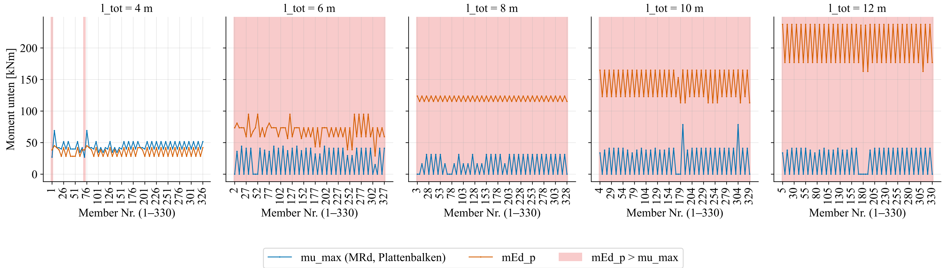
Biege widerstand \mu_{\max} (MRd, Plattenbalken) vs. Bemessungsmoment mEd_p je Member, kategorisiert nach Spannweite (Members_rc_rib_simple_)
